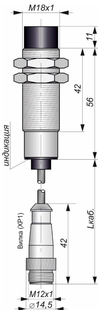
Габаритный чертеж
